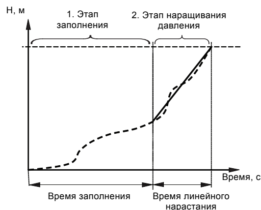
Рис. 31 Этапы заполнения и наращивания давления
