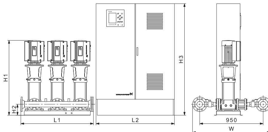
Рис. 59 Размерная схема установки повышения давления Hydro MPC со шкафом управления, смонтированным на полу (исполнение С). Установка повышения давления приведена в качестве примера. Входящие в поставку насосы могут отличаться от показанных на схеме.
