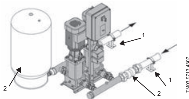
Рис. 3 Пример установки с резиновыми виброподставками и опорами для труб (стандартный объем поставки Grundfos обозначен серым цветом)
