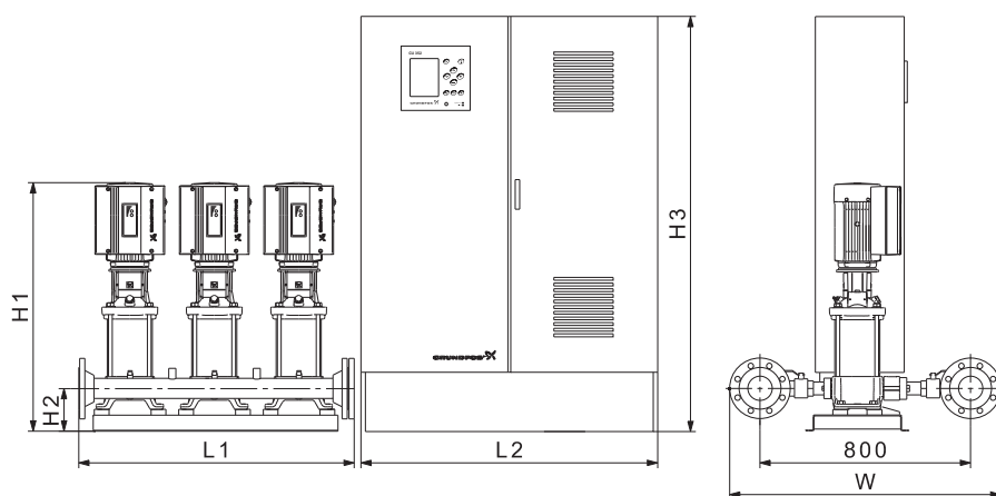
Рис. 53 Размерная схема установки повышения давления Hydro MPC со шкафом управления, смонтированным на полу (исполнение С). Установка повышения давления приведена в качестве примера. Входящие в поставку насосы могут отличаться от показанных на схеме.
